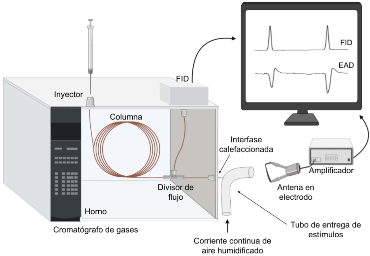
Figura 4. Esquema de Cromatógrafo de Gases (GC) con detector de ionización de llama (FID) acoplado a detector de electroantenografía (EAD).
