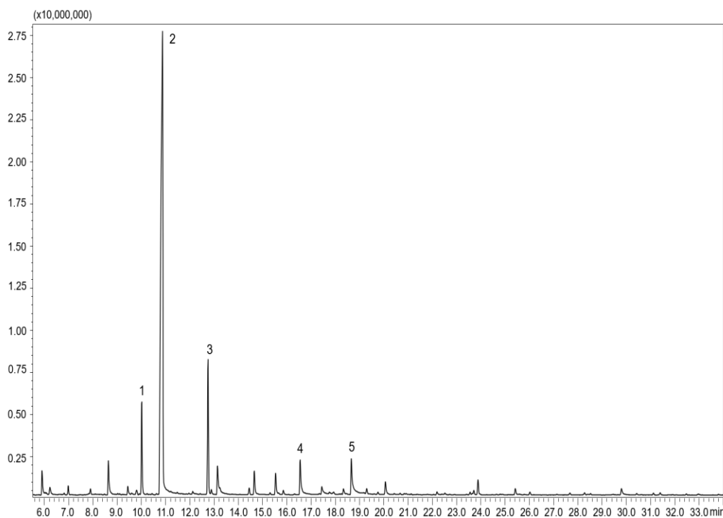
Figura 24. Cromatograma representativo de extracto de VOCs de flores de Malus x domestica variedad Red Chief, obtenidos por GC-MS con columna Rtx-5MS (30 m x 0.25 mm x 0.25 \mu m; Restek). Los números hacen referencia a los compuestos identificados según Tabla 2.
