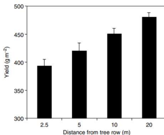
Figura No. 6. Rendimiento de grano de trigo de invierno según la distancia entre filas de árboles en Paulownia, China
