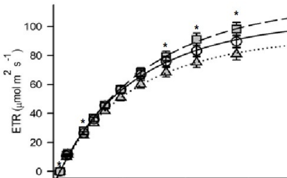
Figura No. 29. Relación entre la radiación fotosintéticamente activa (RFA) y la tasa de transferencia de e^- (ETR) para tres posiciones del experimento
