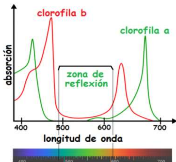
Figura No. 5. Absorción de luz en sus diferentes longitudes de onda por parte de las plantas
