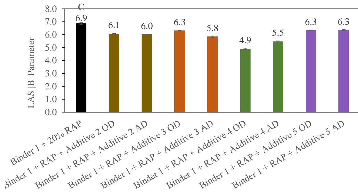
Figure 92. |B| – parameter - Binder 1 + RAP
